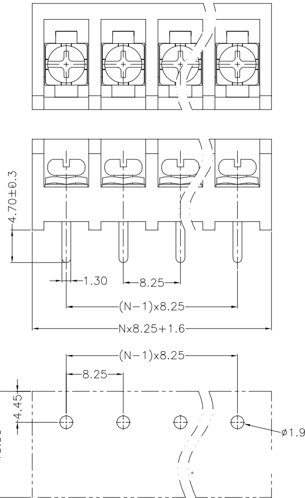
P.C.B.LAYOUT
